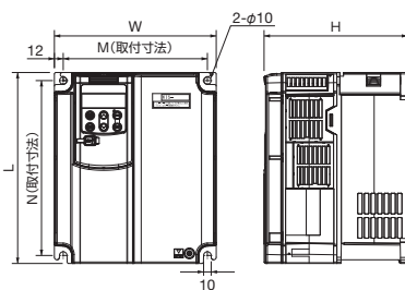
外形図 B: KIS-55F2/KIS-75F2
