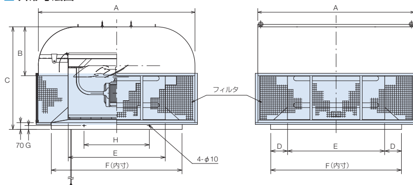
フィルタ (ルーファンに装着時)
